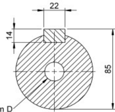
KESİT A-A
